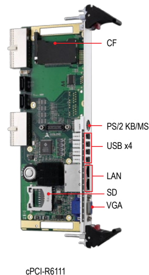
cPCI-R6111
